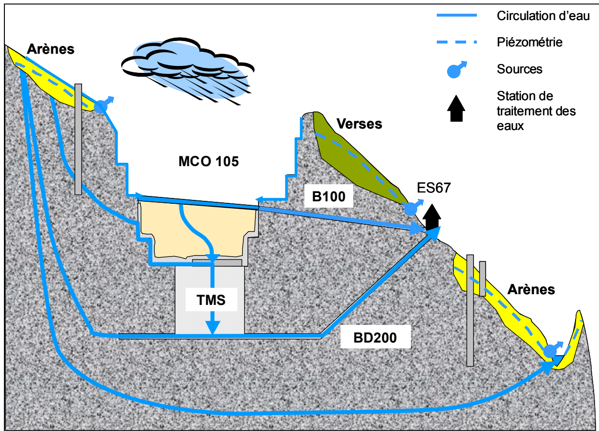
Figure 3 : Transferts d'eau au travers du stockage de résidus de Bellezane (schéma simplifié) (d'après IRSN)
