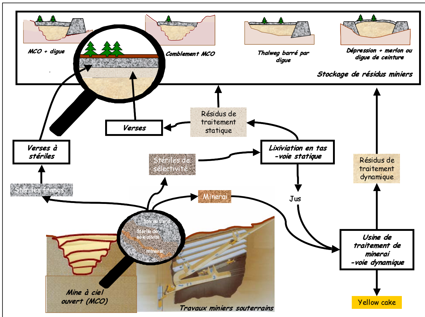
Figure 5 : Traitement du minerai d'uranium (d'après IRSN)
