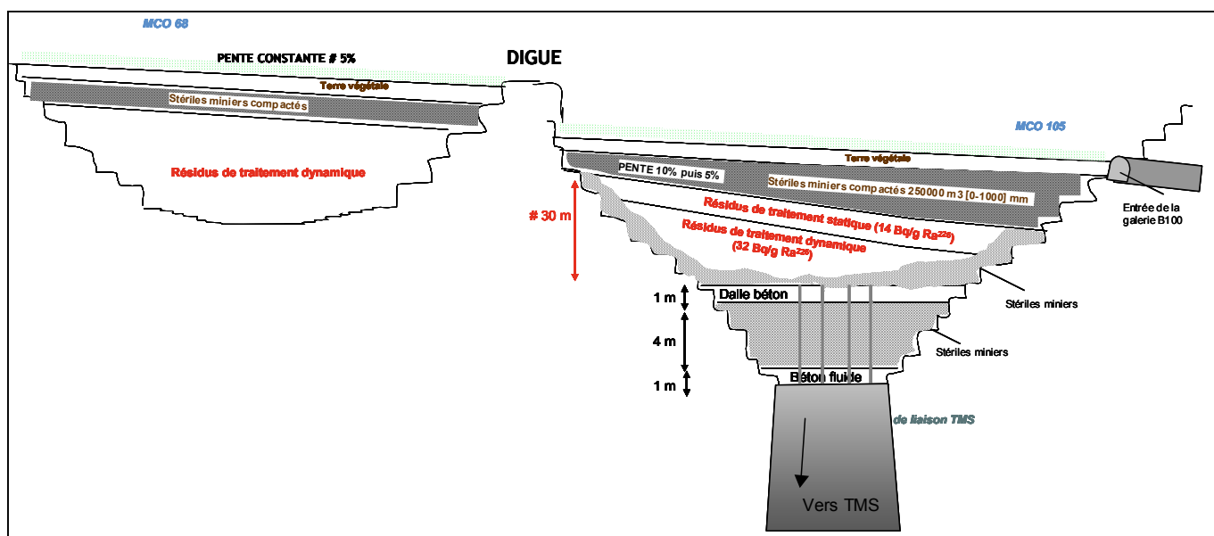
Figure 6 : Coupe schématique du stockage de résidus de Bellezane (d'après IRSN)
