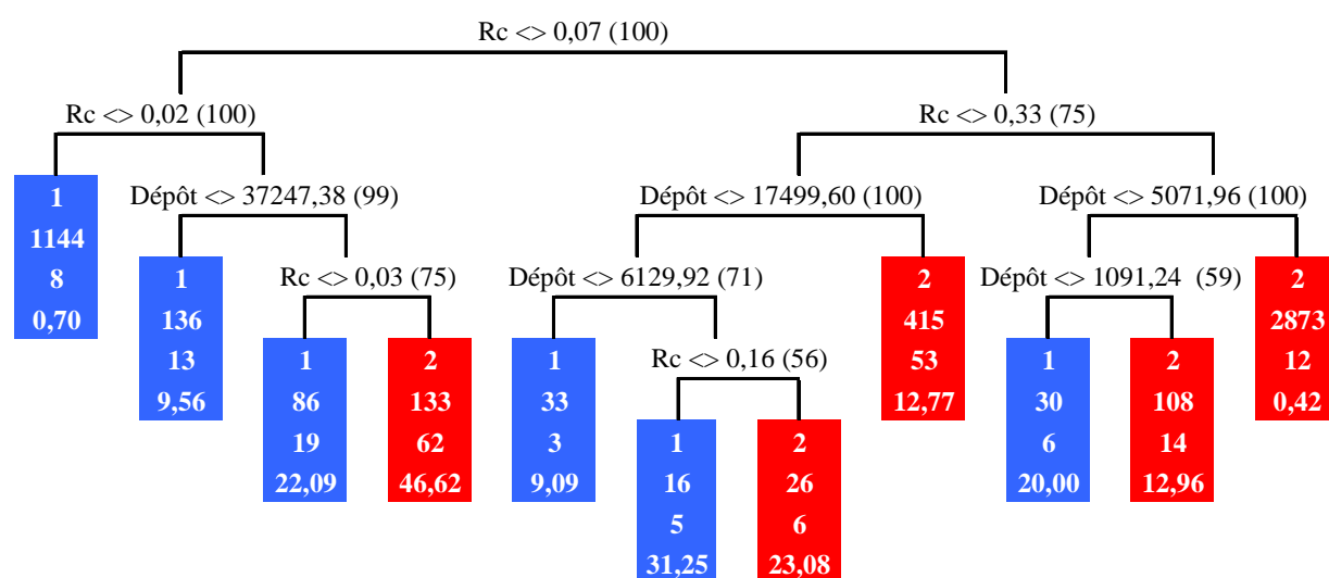
Figure 2 : Arbre de discrimination obtenu pour le scénario de contamination (épinard, ^{90}\text{Sr} )
