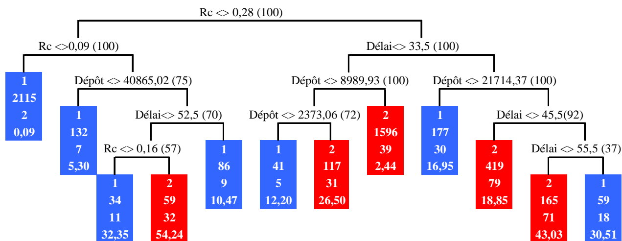
Figure 1 : Arbre de discrimination obtenu pour le scénario de contamination (chou, ^{90}\text{Sr} )
