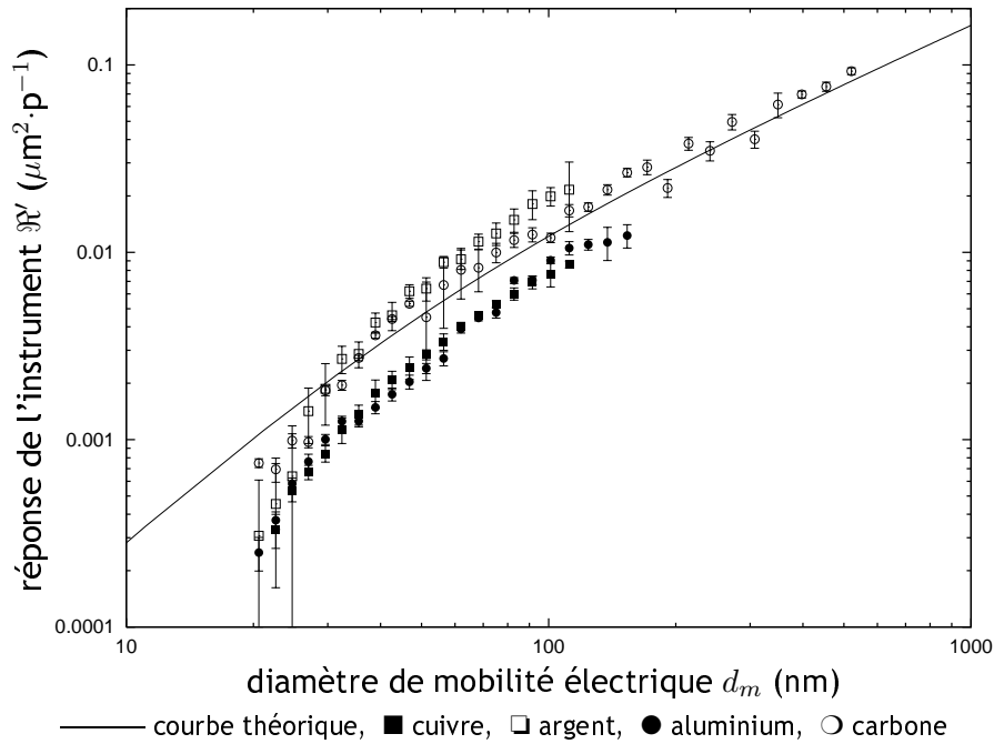
Figure 6.12 - Fonction de réponse du LQ1-DC ( \mathcal{R} = C_{S_a}/C_N ) établie sur des aérosols monodispersés issus du banc d'essais CAIMAN pour différentes natures d'électrodes - données LQ1-DC/CNC
