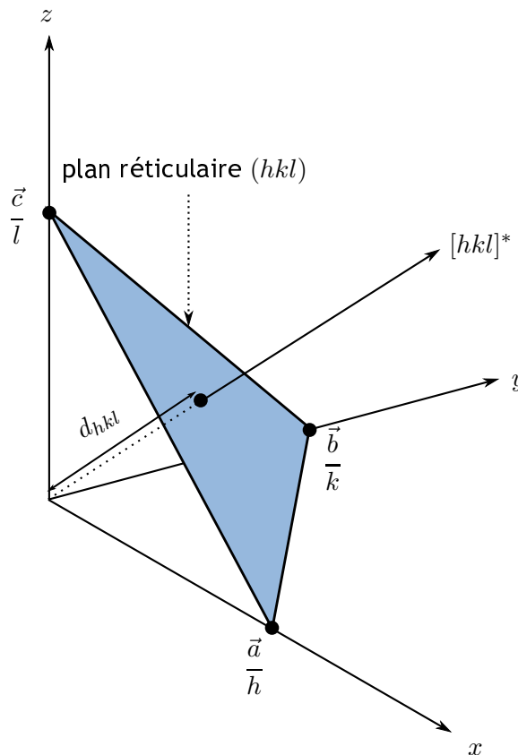
Figure D.1 - Représentation schématique de la distance interréticulaire d_{hkl}
