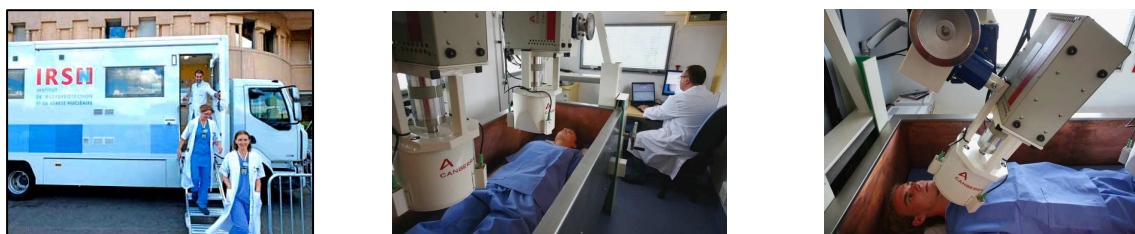
Figure 7 - Vues du laboratoire mobile d'anthroporadiamétrie LMA
