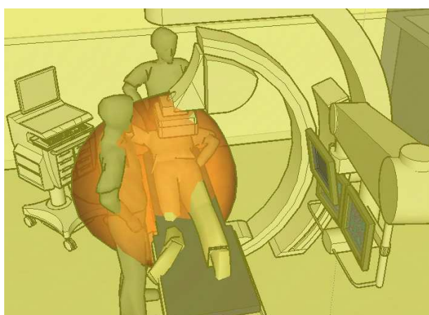
Figure 27 - Zonage tridimensionnel de la salle monoplan lors d'une vertébroplastie
