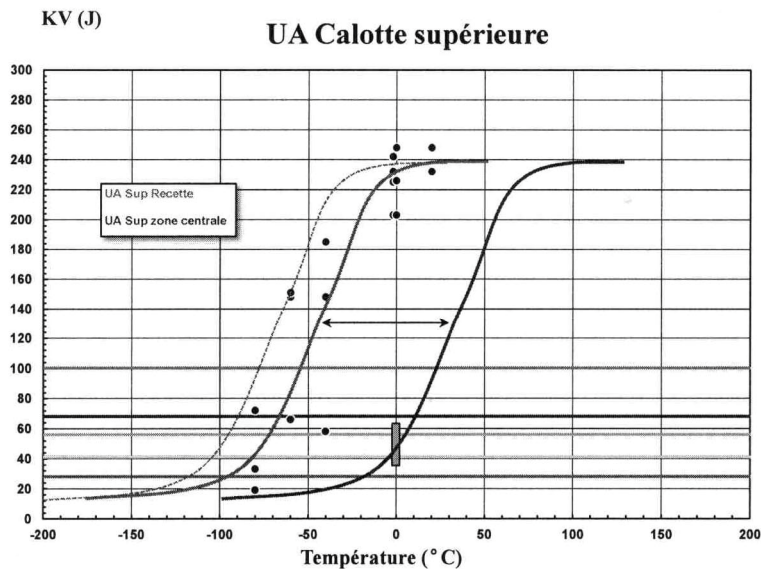
Figure 26 : Calotte UA. Évaluation de la transition de résilience entre zone de recette et 1/4 épaisseur tête
