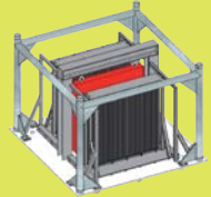
Dispositif des expériences où un matériau de forte épaisseur est positionné sous forme d'écran entre deux réseaux de crayons d' UO_2 avec lesquels il est en interaction. Matériaux testés : fer, nickel, zirconium, aluminium, plomb, cuivre ou béton pour différentes teneurs en eau (3 %, 6 %, 9 %) et pour des épaisseurs de l'écran variant entre 5 cm et 30 cm.
