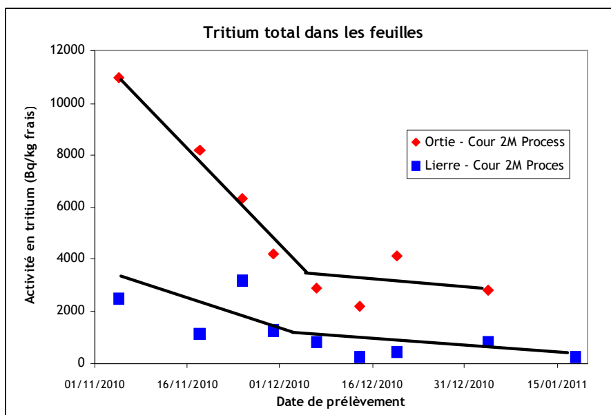
Figure 2 - Évolution au cours du temps de l'activité en tritium mesurée entre le 5 novembre 2010 et le 18 janvier 2011 dans des feuilles d'orties et de lierre prélevées dans la cour de 2M Process, respectivement à deux mètres et moins de 10 mètres du bâtiment contaminé
