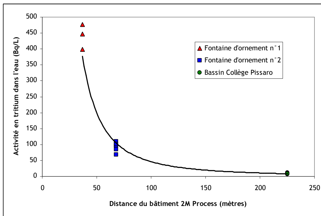
Figure 1 - Évolution de l'activité en tritium mesurée entre le 18 novembre 2010 et le 18 janvier 2011 dans les eaux de surface en fonction de la distance du site de 2M Process
