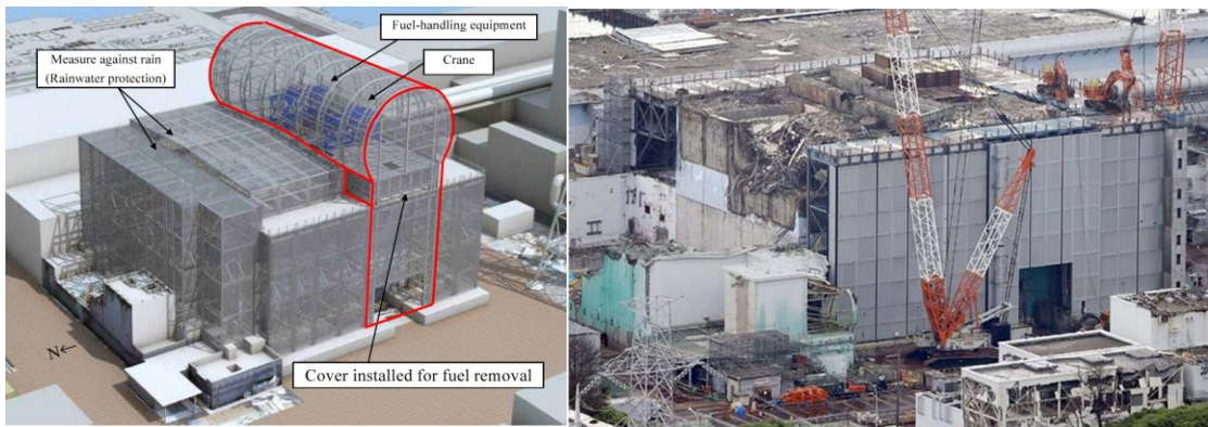
Source TEPCO - Projet de couverture du bâtiment réacteur 3 et avancement des travaux correspondant à l'été 2013
