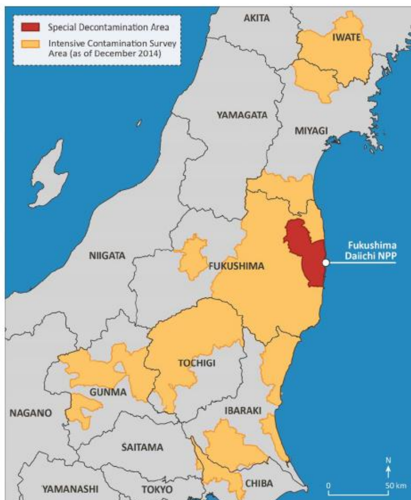
Figure 2 : Localisation de la « Special Decontamination Area - SDA » (en rouge) et la « Intensive Contamination Survey Area - ICSA » mises en place par les autorités japonaises fin 2011. 2
