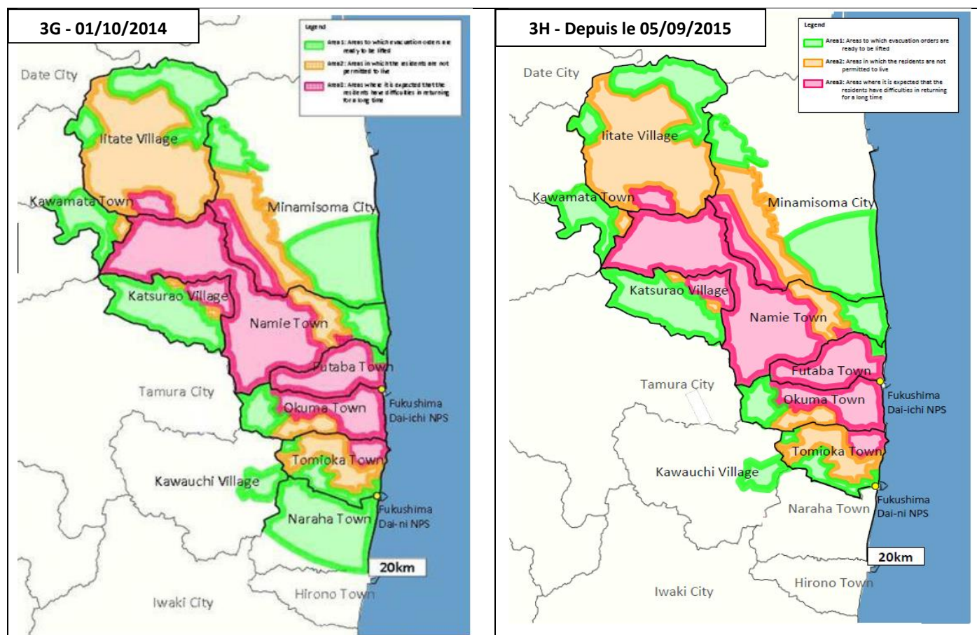
Figure 3 : Evolution du zonage de la « Special Decontamination Area » entre avril 2012 et septembre 2015.
