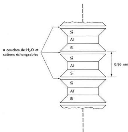
FIGURE 2.3.5: Schéma de la structure de la montmorillonite, d'après Lambe (1953) cité par Holtz & Kovacs (1981)
