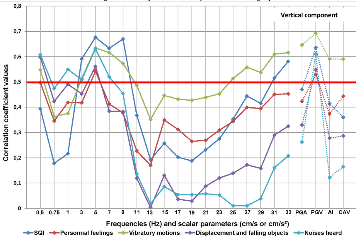
Figure 24: Coefficient de corrélation R entre les paramètres instrumentaux et macrosismiques dans des cercles de 10km autour des stations accélérométriques pour les trois séismes confondus. a) Corrélations avec la résultante des deux composantes horizontales. b) Corrélations avec la composante verticale. La partie droite de la figure montre les coefficients de corrélation entre les paramètres macrosismiques et les paramètres instrumentaux scalaires (PGA, PGV, AI, CAV). La partie gauche de la figure montre les coefficients de corrélation entre les paramètres macrosismiques et les spectres de réponse entre 0.5 et 33Hz. La ligne rouge est la corrélation seuil de R=0.5 à partir de laquelle la corrélation devient significative.
