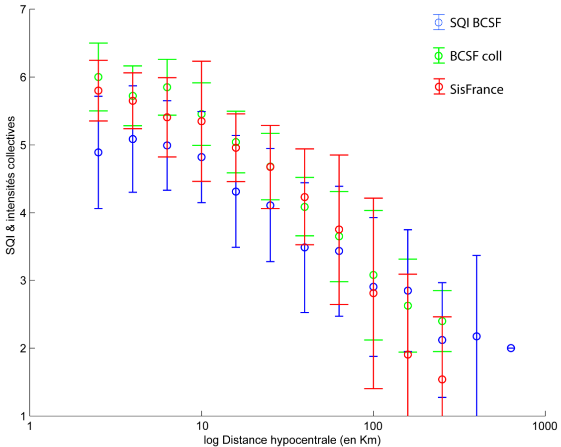
Figure 3: Intensité moyenne estimée par classe de distance hypocentrale pour le séisme de Rambervillers ( 22/03/2003, Mw=4.8, h=12km) à partir des intensités collectives SisFrance et BCSF et SQJ. Les barres verticales sont les barres d'erreur à \pm 1\sigma
