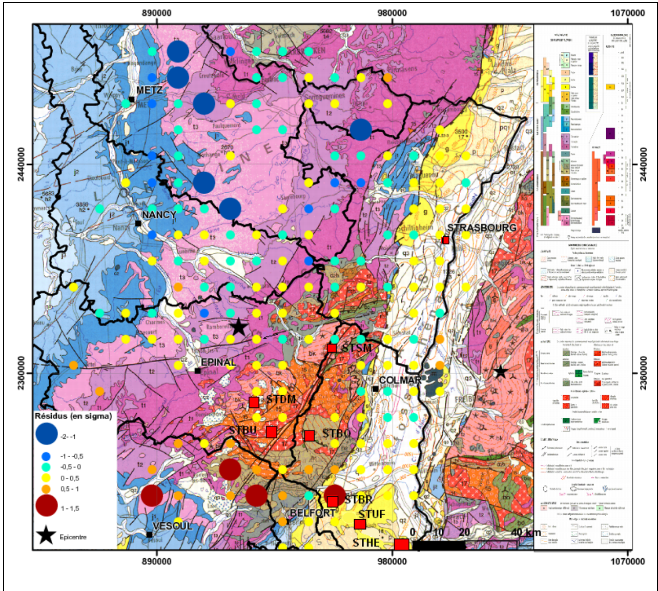
Figure 18: Carte de répartition des résidus (SQI-SQI_{mod}) / \sigma_{mod} pour le séisme de Rambervillers. Les cercles jaune à rouge sont les résidus positifs tandis que les cercles bleus figurent les résidus négatifs. Les stations accélérométriques sont figurées par des carrés rouges à bordure noire. Pour la clarté de la figure les cercles de 10km autour des stations n'ont pas été représentés.
