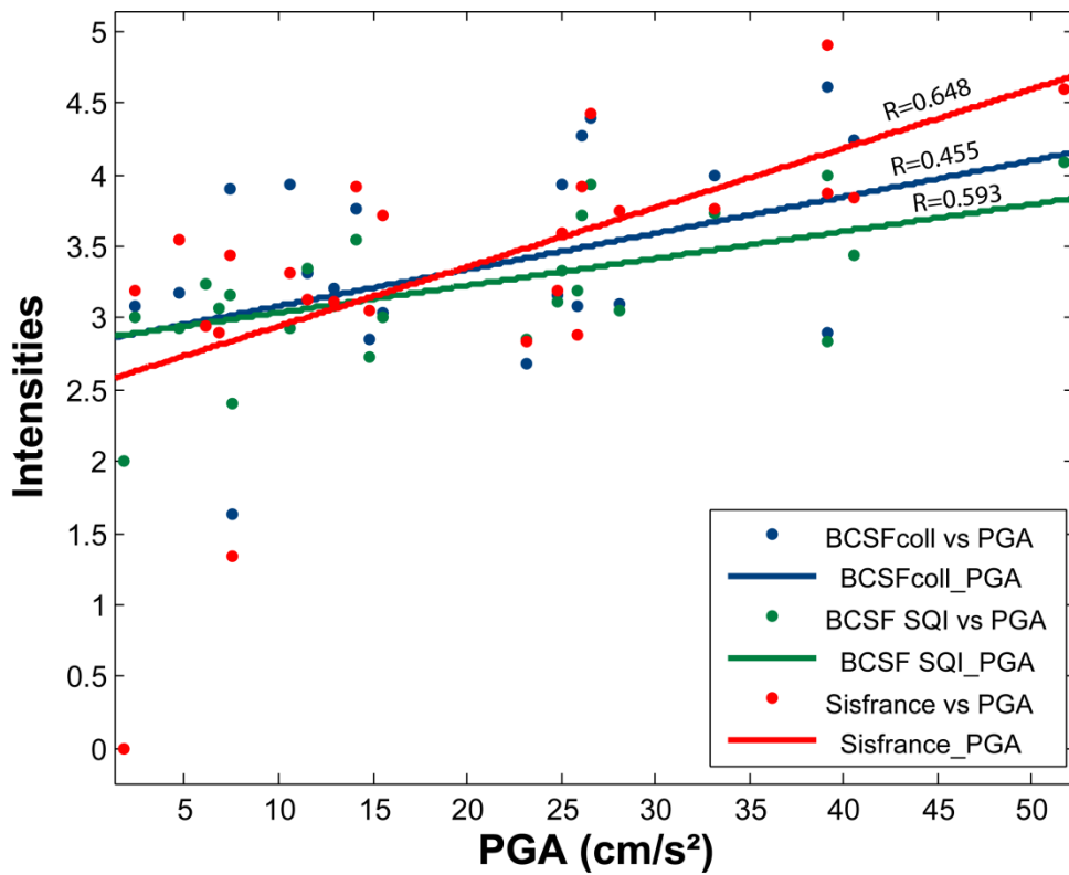
Figure 27: Intensités collectives BCSF (BCSFcoll), SisFrance, et SQI en fonction du PGA 10km autour des stations accélérométriques avec droites de corrélation entre les intensités et les PGA
