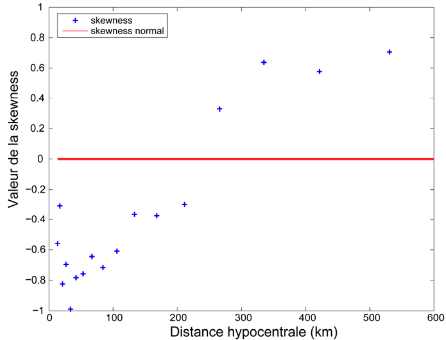
Figure 15: Skewness de la distribution des SQI agrégées par commune en fonction de la distance hypocentrale pour le séisme de Rambervillers. La ligne rouge présente la valeur de la skewness d'une distribution normale. Dans le cas présent les valeurs de la skewness en fonction de la distance hypocentrale montrent les données sont biaisées.
