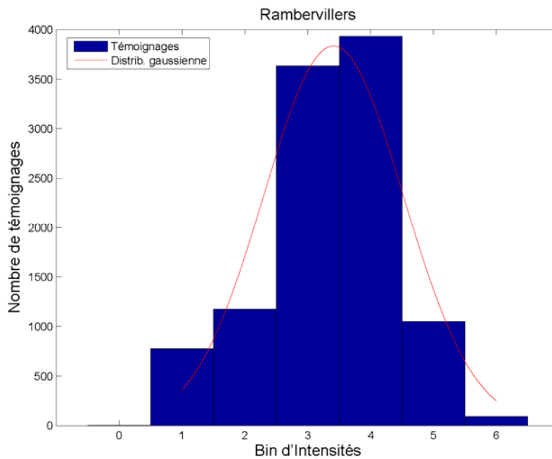
Figure 5: Répartition spatiale des SQI selon leurs valeurs pour le séisme de Rambervillers et histogramme du nombre de témoignage en fonction des valeurs des SQI. Les étoiles rouges représentent les epicentres des séismes. Les points bleus figurent les témoignages individuels collectés pour les trois séismes. Les triangles rouges représentent les stations accélérométriques du RAP qui ont enregistré les séismes et les cercles rouges sont des zones de 10km de rayon autour des stations.
