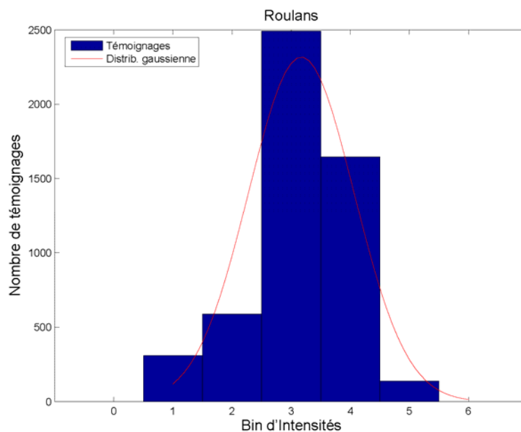
Figure 6: Répartition spatiale des SQI selon leur valeur pour le séisme de Roulans et histogramme du nombre de témoignage en fonction des valeurs des SQ. Les étoiles rouges représentent les epicentres des séismes. Les points bleus figurent les témoignages individuels collectés pour les trois séismes. Les triangles rouges représentent les stations accélérométriques du RAP qui ont enregistré les séismes et les cercles rouges sont des zones de 10km de rayon autour des stations.
