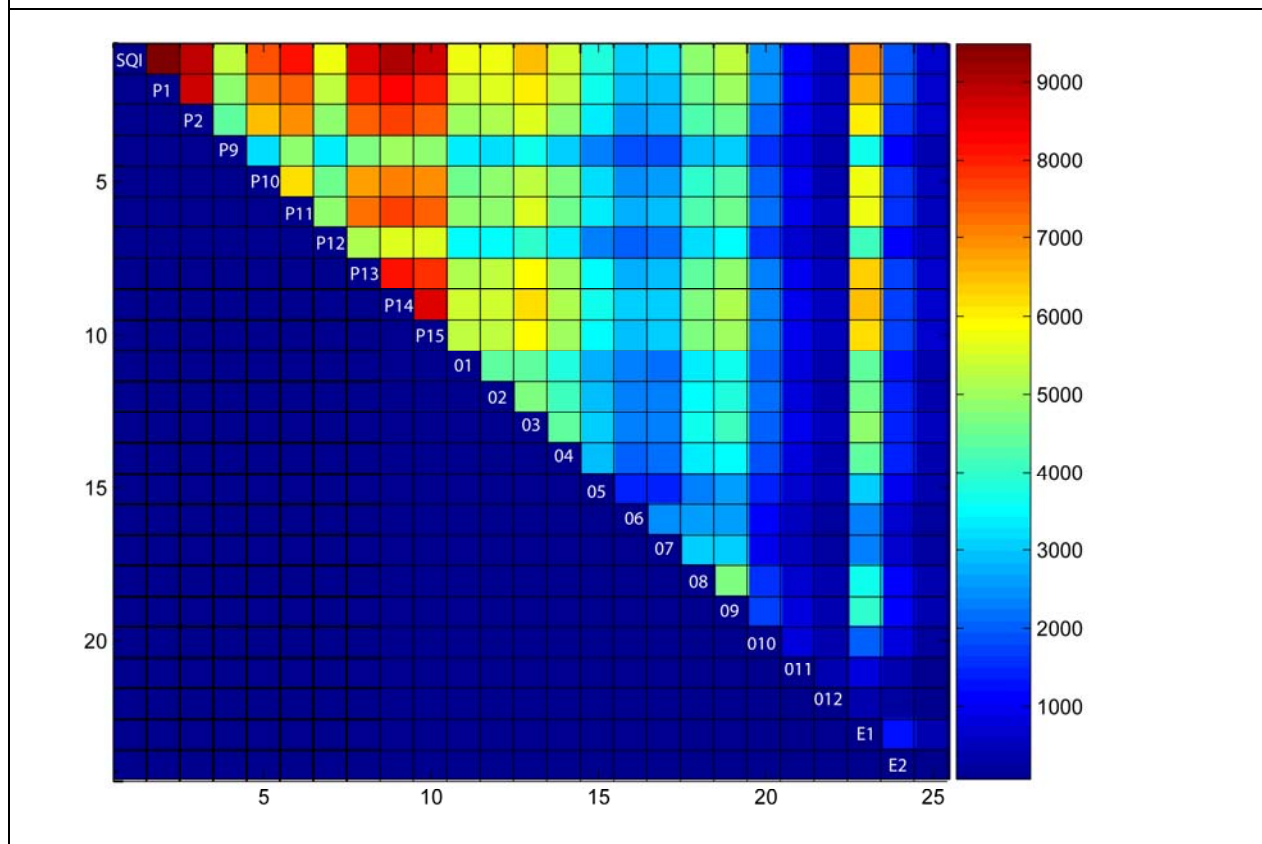
Figure 8: a) Matrice de corrélation réduite pour le séisme de Rambervillers. Chaque carré correspond à la valeur de la corrélation entre les réponses à deux questions. Les traits pleins noirs délimitent les champs de questions retenus car présentant des corrélations fortes entre les questions, les traits pointillés blancs délimitent les corrélations entre les différents champs de questions. b) Matrice du nombre de témoignages à partir desquels sont calculées les corrélations entre les réponses aux questions. Chaque carré correspond au nombre de témoignage communs à deux questions
