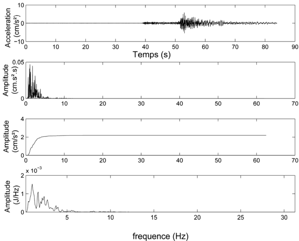
Figure 30: Pour la station STHE, signal accélérométrique enregistré lors du séisme de Rambervillers, spectre de Fourier, spectre d'accélération et densité spectrale de puissance
