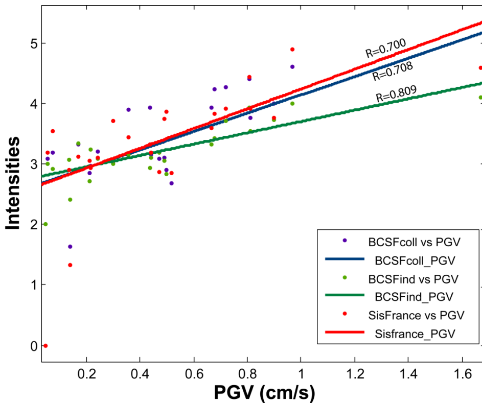
Figure 28: Intensités collectives BCSF (BCSFcoll), SisFrance, et SQI (BCSFfind) en fonction du PGV 10km autour des stations accélérométriques avec droites de corrélation entre les intensités et les PGV
