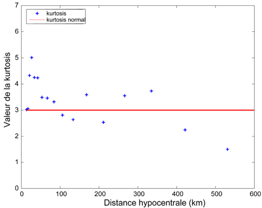
Figure 16: Kurtosis de la distribution des SQI agrégées par communes en fonction de la distance hypocentrale pour le séisme de Rambervillers La ligne rouge présente la valeur de la kurtosis d'une distribution normale. Dans le cas présent les valeurs de la kurtosis en fonction de la distance hypocentrale montrent les données sont biaisées.
