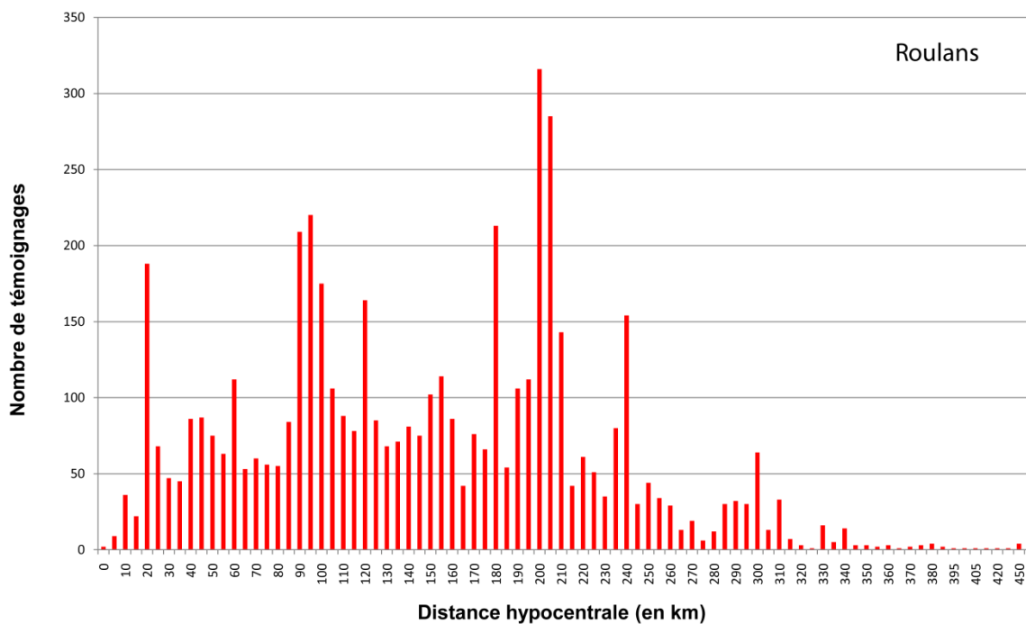
Figure 13: Nombre de témoignages en fonction de la distance hypocentrale pour le séisme de Roulans
