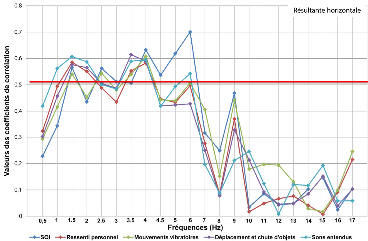
Figure 31: Corrélations entre les paramètres macrosismiques et la résultante horizontale de la densité spectrale de puissance
