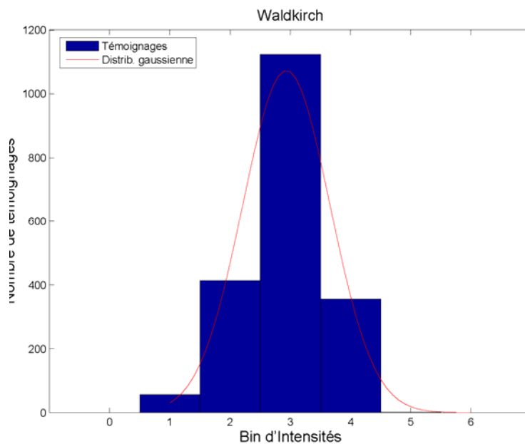
Figure 7: Répartition spatiale des SQJ selon leur valeur pour le séisme de Waldkirch et histogramme du nombre de témoignage en fonction des valeurs des SQJ. Les étoiles rouges représentent les épicentres des séismes. Les points bleus figurent les témoignages individuels collectés pour les trois séismes. Les triangles rouges représentent les stations accélérométriques du RAP qui ont enregistré les séismes et les cercles rouges sont des zones de 10km de rayon autour des stations.
