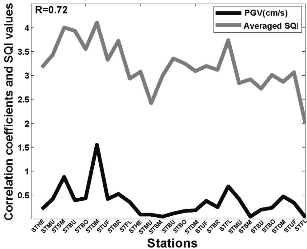
Figure 23: Signification de la corrélation à partir d'une paire de paramètres instrumentaux (PGV) et macrosismiques (<SQI>). La courbe grise représente la moyenne des SQI sur les cercles de 10km autour de chaque station accélérométrique pour chacun des 3 séismes La courbe noire représente le PGV horizontal correspondant au PGV du signal horizontal portant le maximum du PGA (voir section 3.3.1) à chaque station Une régression linéaire entre les <SQI> et les PGV donnent la corrélation de R=0.72 , montrée sur la Figure 29: Corrélation entre les paramètres macrosismiques et la composante horizontale du mouvement du sol qui porte le PGA maximum. Corrélations des paramètres macrosismiques avec le PSA (à gauche) et avec les paramètres scalaires du mouvement du sol (à droite)Figure 29.
