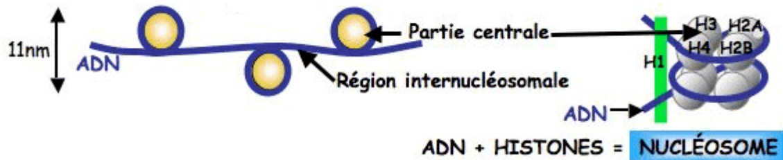
Figure I-13 : Nucléosomes [WEB03].
